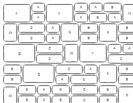
52 pièces ayant 7 formats, Dimensions du système: 1.16 x 0.80 = 0,9 m 2
